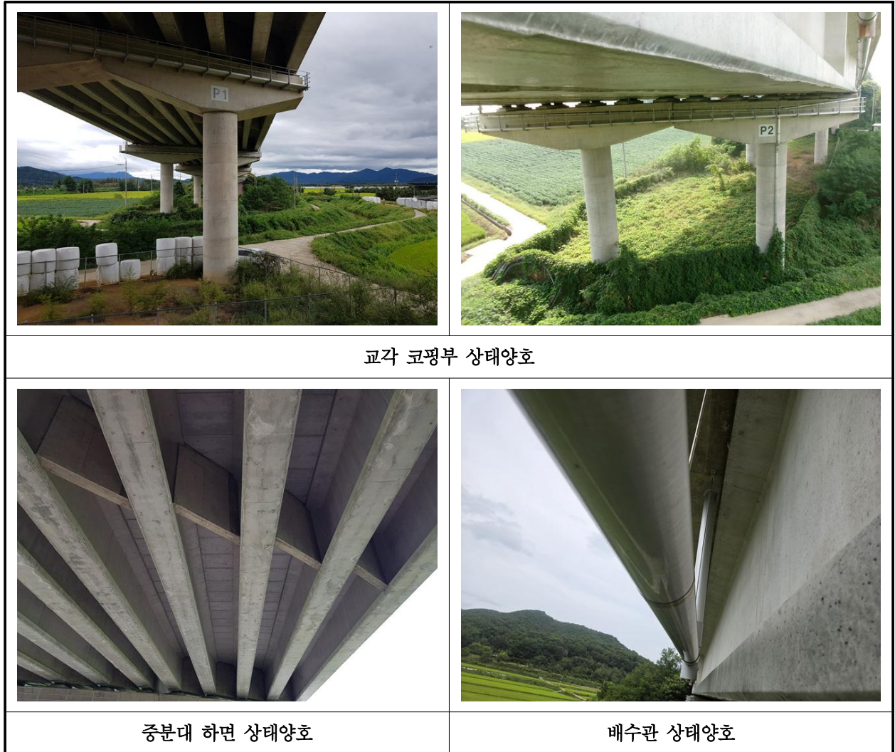
【사진 4.3.54】 교량의 공중이용시설 10대 위험요소 손상현황
